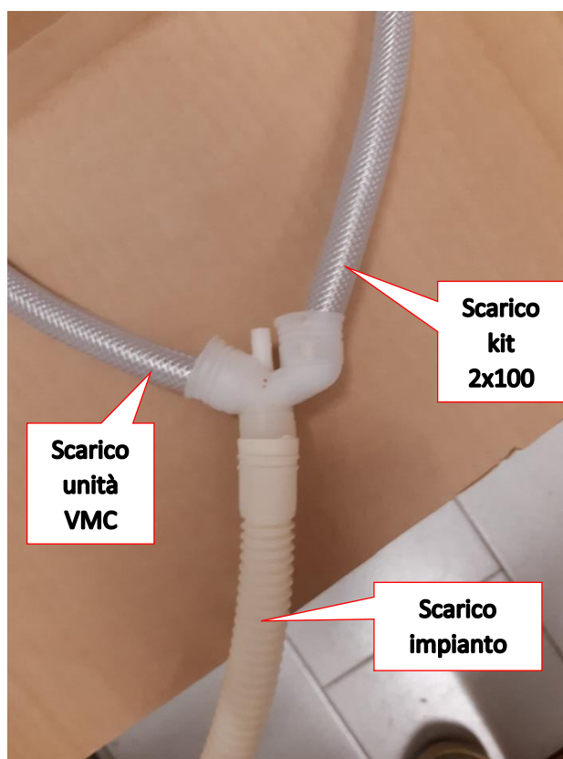
Esempio di collegamento scarichi
