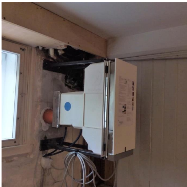
Tubi rigidi per ripresa e per espulsione In questo caso i tubi sono interni allo spessore del muro
