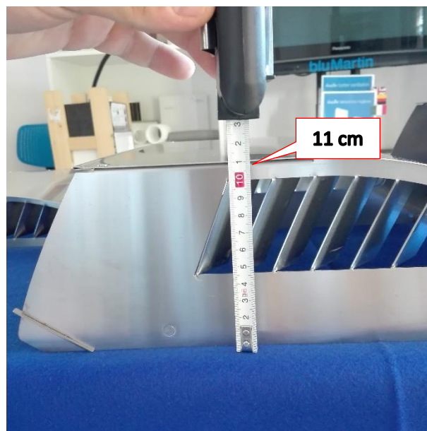
da 35 a 40 cm – sporgenza guscio 11 cm
